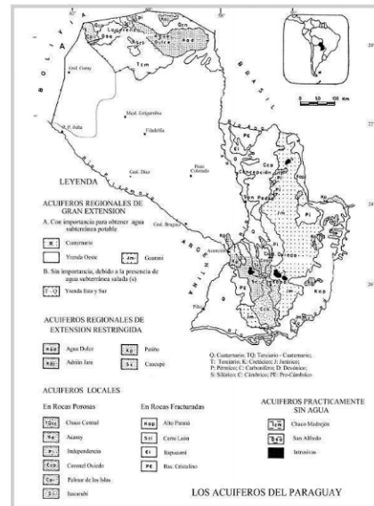
Figura 5. Acuíferos del Paraguay
