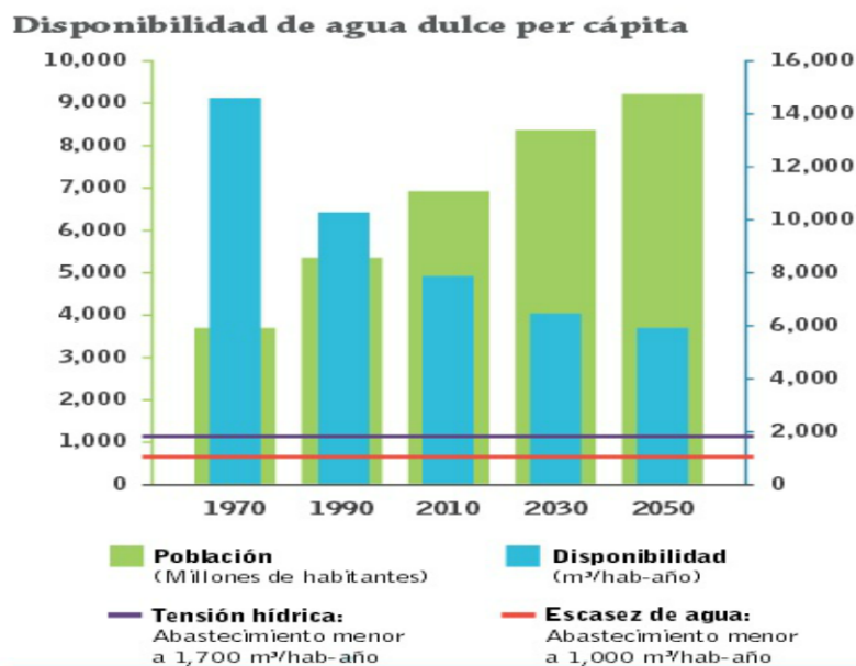
Figura 1. Disponibilidad de agua dulce per cápita
