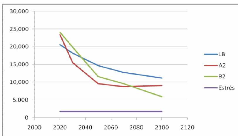
Figura 12. Variación de la disponibilidad per cápita (m3/hab/año)
