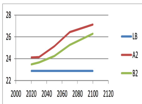
Figura 8. Variación de la Temperatura (°C)
