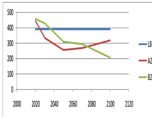
Figura 11. Variación de la escorrentía en (mm/año)
