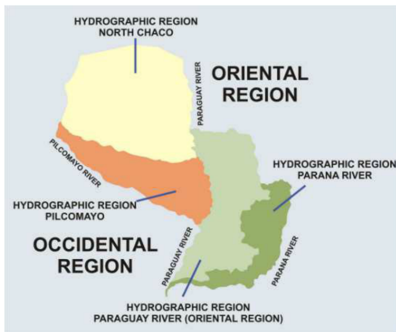
Figura 6. Regiones Hidrográficas (elaboración propia)
