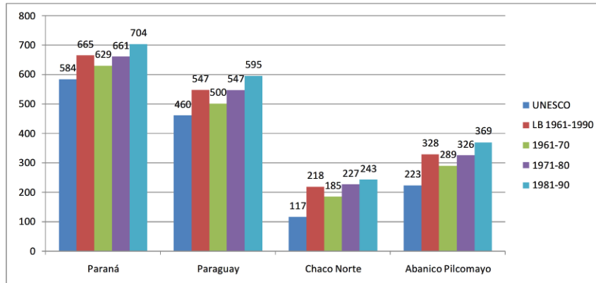
Figura 7. Escorrentía (Run Off) en milímetros por Región Hidrográfica
