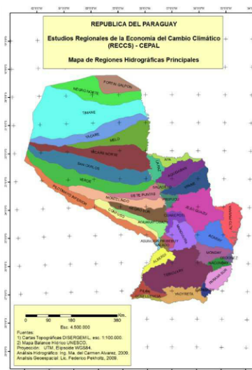
Figura 3. Cuencas del Paraguay
