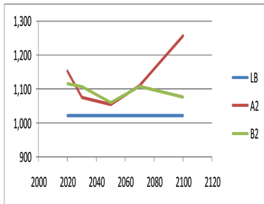
Figura 10. Variación de la Evapotranspiración en (mm/año)
